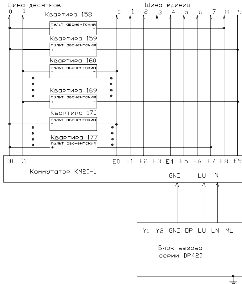
Рис.1 Вариант схемы подключения КМ20-1
