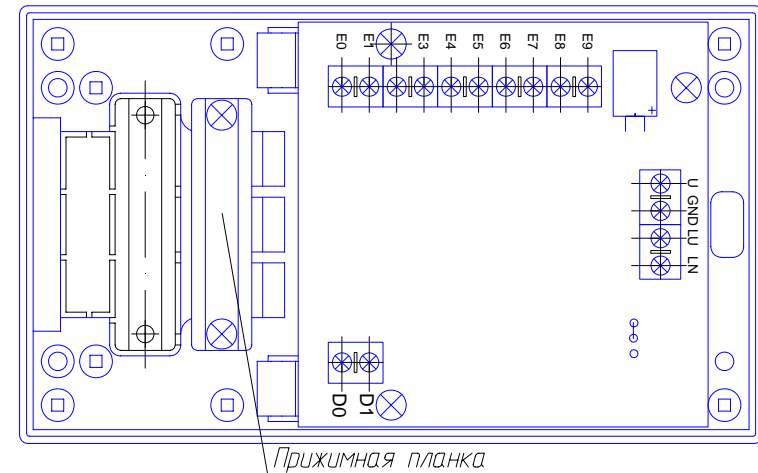
Рис.2 Внешний вид изделия со снятой крышкой.
